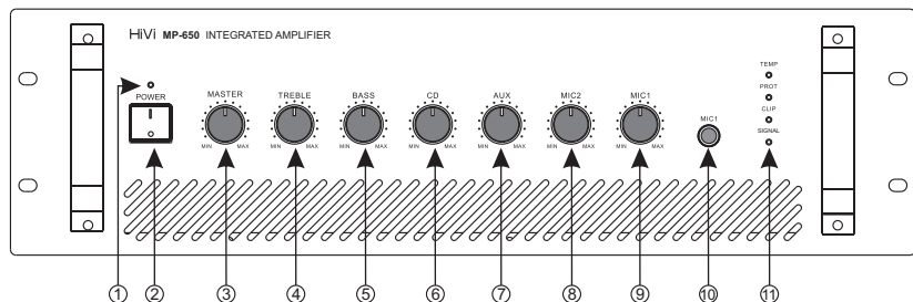
前面板
